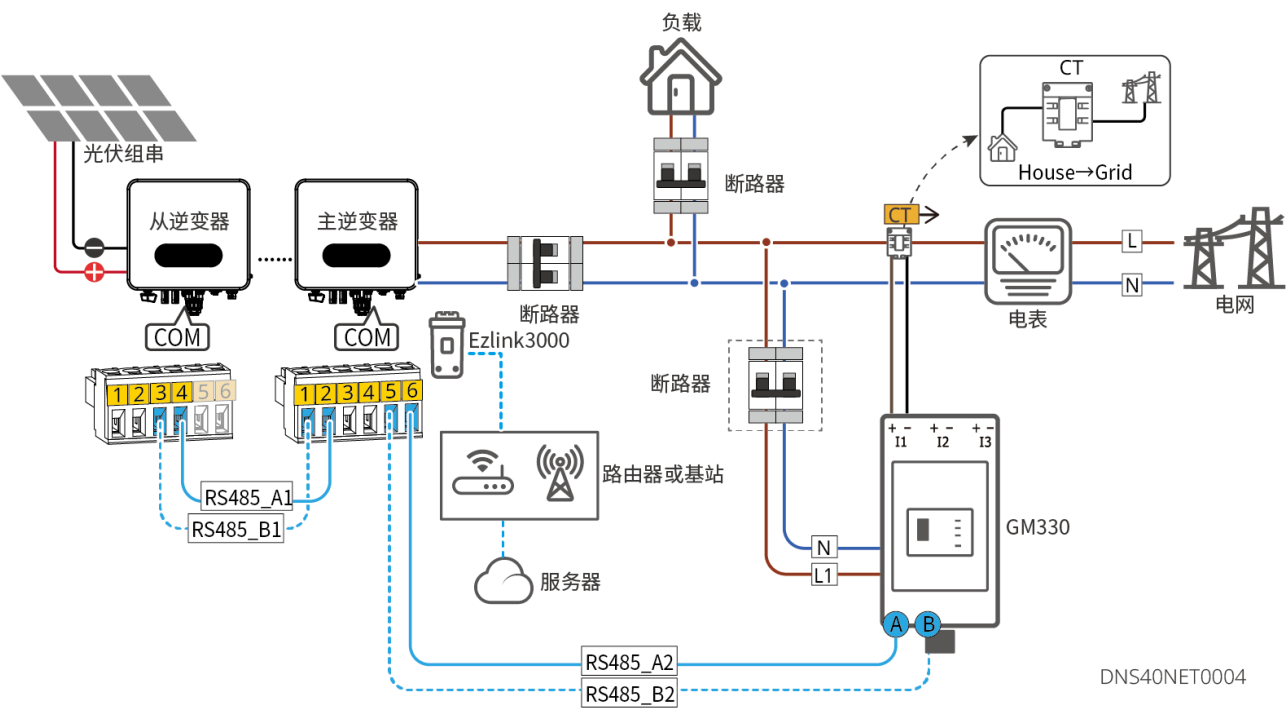
多机功率限制组网方案（GM330+Ezlink3000）
